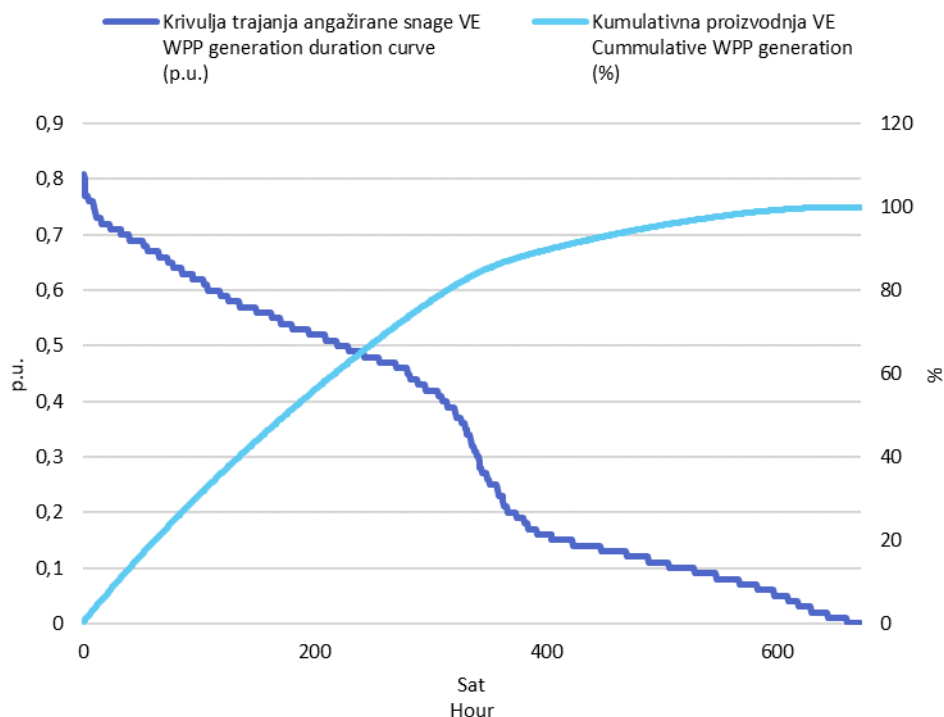
Slika 3 Krivulja trajanja angažirane snage svih VE i kumulativna proizvodnja VE u veljači 2023. godine u jediničnim vrijednostima
